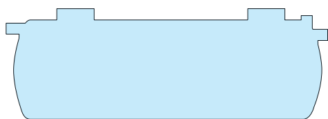
MIRI OAS-4
