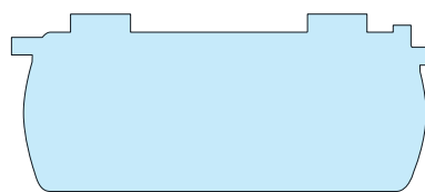
MIRI OAS-3
