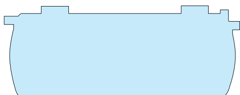
MIRI OAS-6
