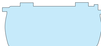
MIRI OAS-5
